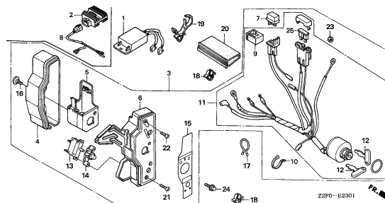
コントロールボックス (2)
