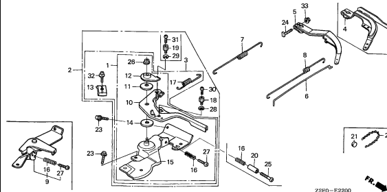
コントロールボックス (2)
