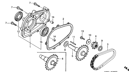
リダクション (1)
