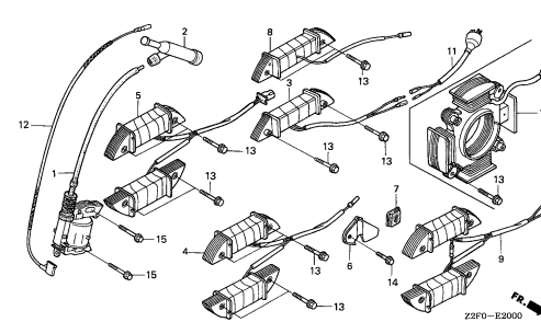
コントロール (2)
