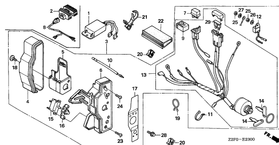
コントロールボックス (1)
