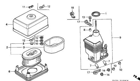
エアークリーナー(4)
