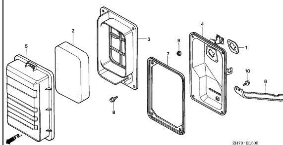
エアークリーナー(6)
