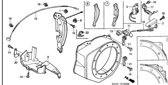
ファンカバー
