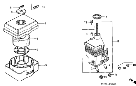
エアークリーナー(6)
