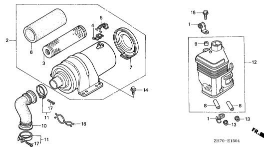
エアークリーナー(5)
