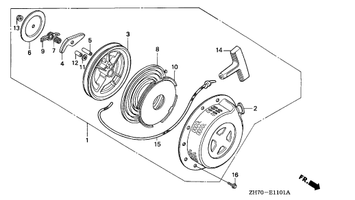
リコイルスターター(2)
