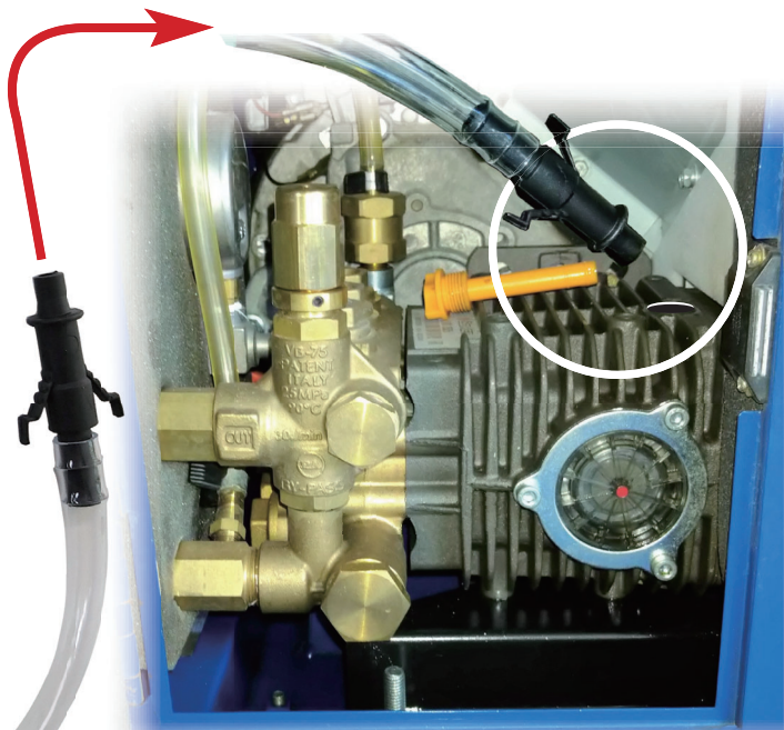
▲高圧洗浄機JC-1513DPN+ ポンプ部
