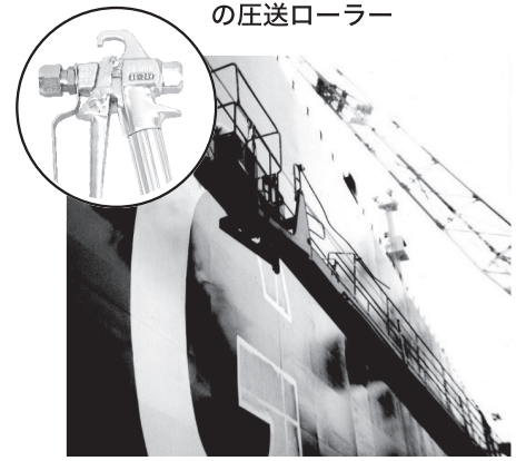
重防蝕塗料のエアレス吹き
