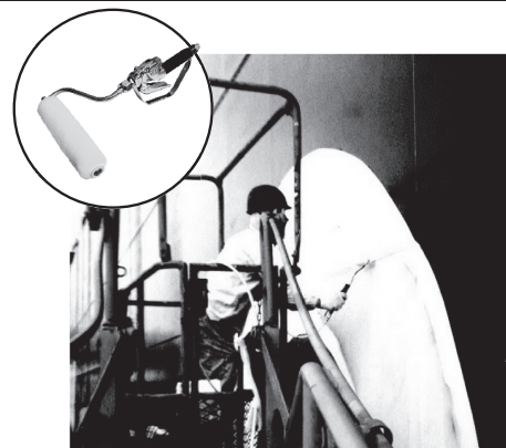
超高粘度塗料・特殊接着剤 の圧送ローラー
