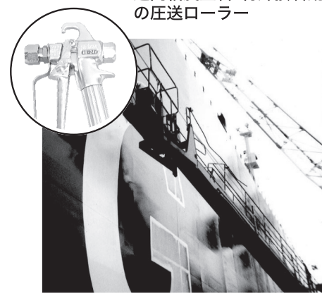
重防蝕塗料のエアレス吹き
