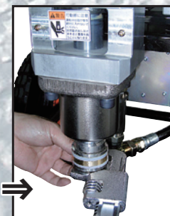
③ 吐出弁を外す
