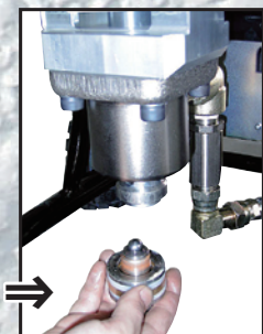
④ パッキンを外し、交換する ※ 逆の順序で組み立てる
