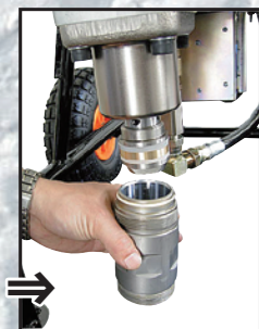
② シリンダーを抜く
